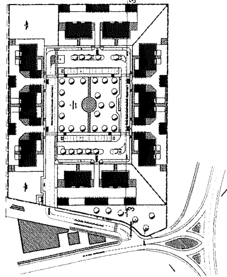
CALCOLO VOLUME EDIFICI • PERTINENZE DA EDIFICARE
